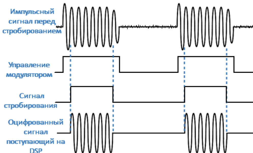
Рисунок 18 – Временная диаграмма режима программного стробирования
