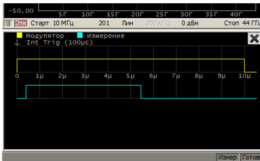
Рисунок 20 – Пример временной диаграммы для настройки импульсного режима
