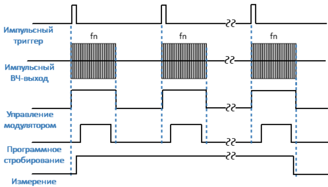
Рисунок 24 – Измерение в одной точке развертки в узкополосном режиме
