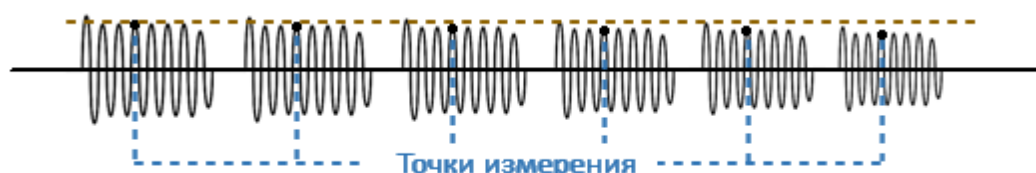
Рисунок 28 – Пример изменения коэффициента усиления от импульса к импульсу
