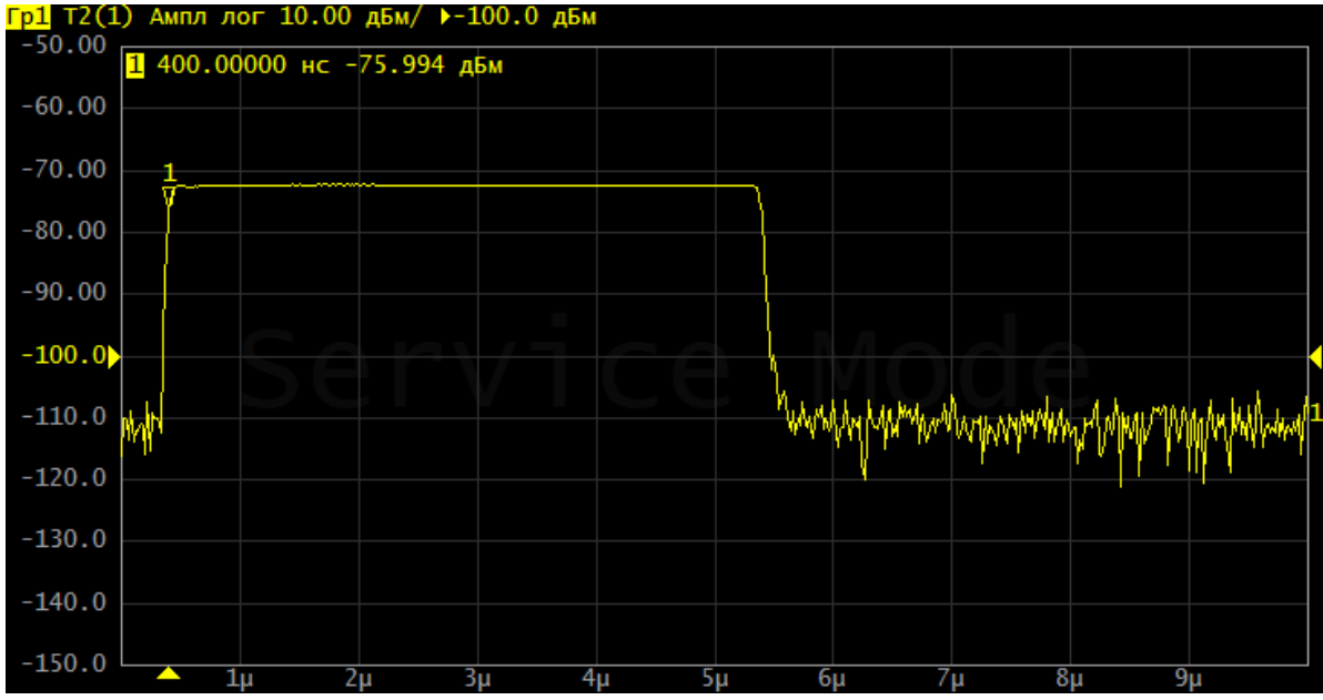
Рисунок 19 – Определение суммарной задержки модулятора и задержки в цепях подключения ИУ
