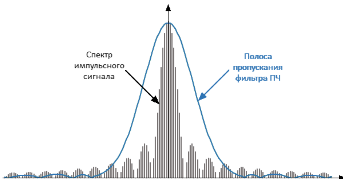
Рисунок 5 – Широкополосное детектирование
